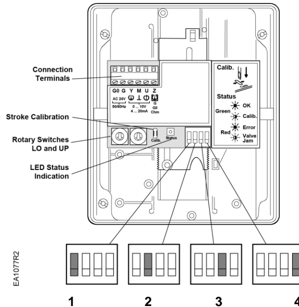
Figure 23. SKB/C62UA.
